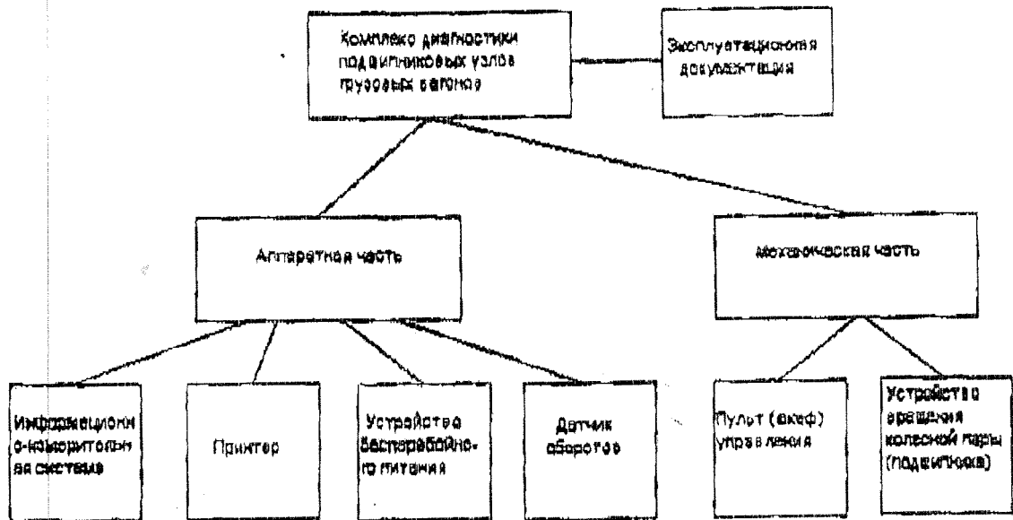
Рисунок 1. Обобщенная структурная схема комплекса вибродиагностики подшипников буксовых узлов колесных пар
