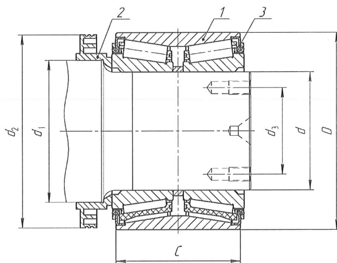
Рисунок 8 – Вариант исполнения с передней крышкой с четырьмя болтами, с заглушкой
