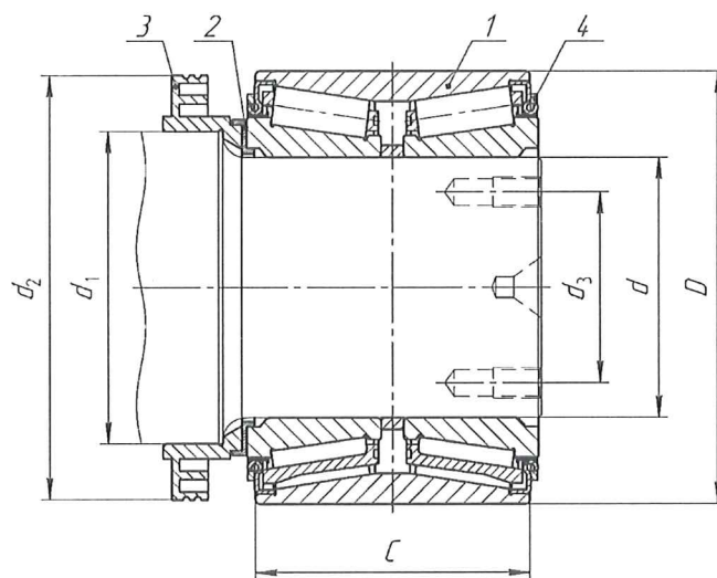
Рисунок 7 – Вариант исполнения с лабиринтным кольцом и полимерной прокладкой без передней крышки
