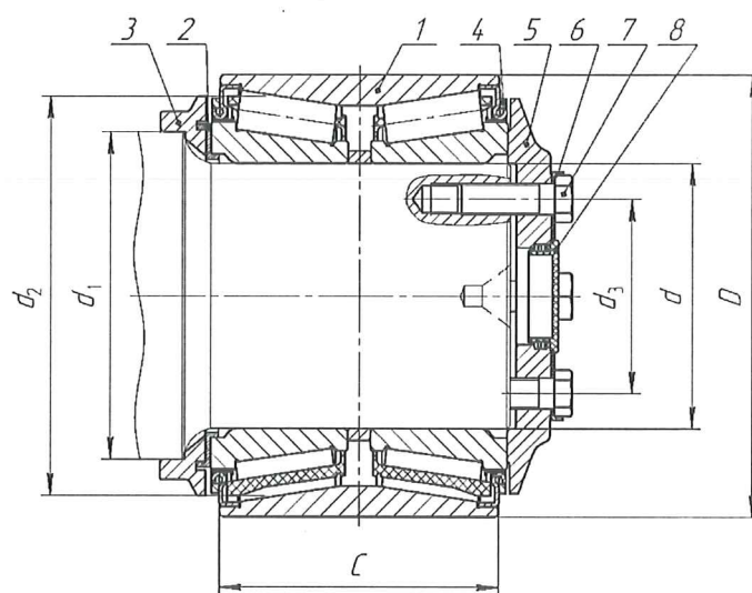
Рисунок 4 – Вариант исполнения с передней крышкой без заглушки, с четырьмя болтами
