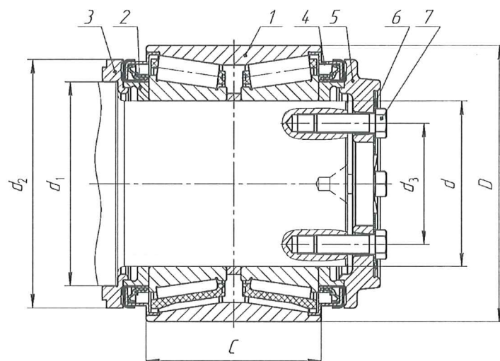
Рисунок 4 – Вариант исполнения с передней крышкой без заглушки, с четырьмя болтами
